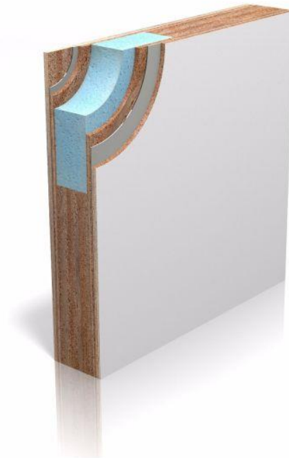
Isolatiedeur
